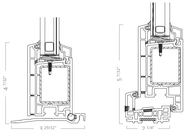
ADA Sill
