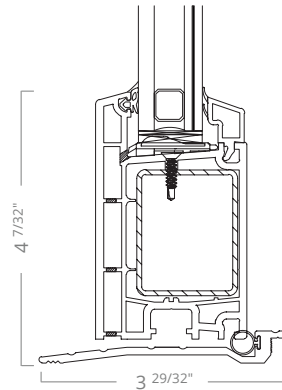
ADA Sill
