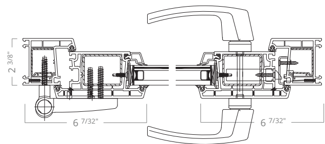
Terrace Door w/o Flange
