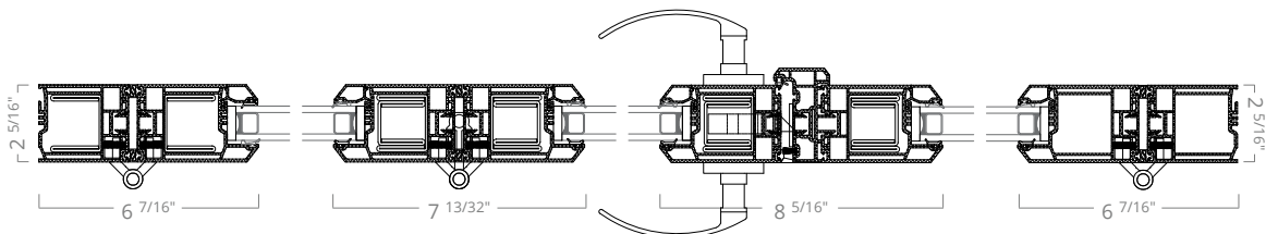
Standard Jamb
