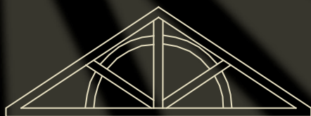
Arched Fan Option 1
