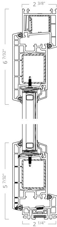
Terrace Door w/o Flange
